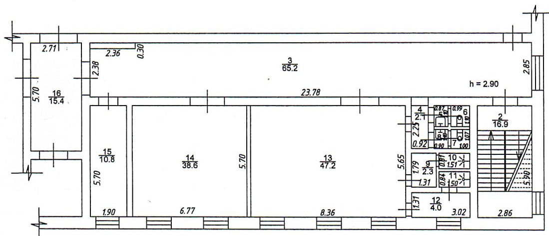
Этаж 2
