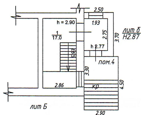
Этаж 1
